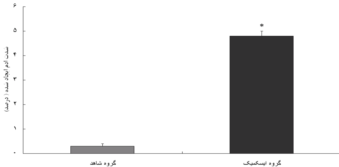
نمودار ۶. شدت ادم ایجاد شده در نیمکره ایسکمیک (چپ) مغز در حیوانات گروه شاهد (n=8) و گروه ایسکمیک (n=8)، ۲۴ ساعت پس از وقوع ایسکمی مغزی (* نسبت به گروه شاهد p < 0.05 ).
