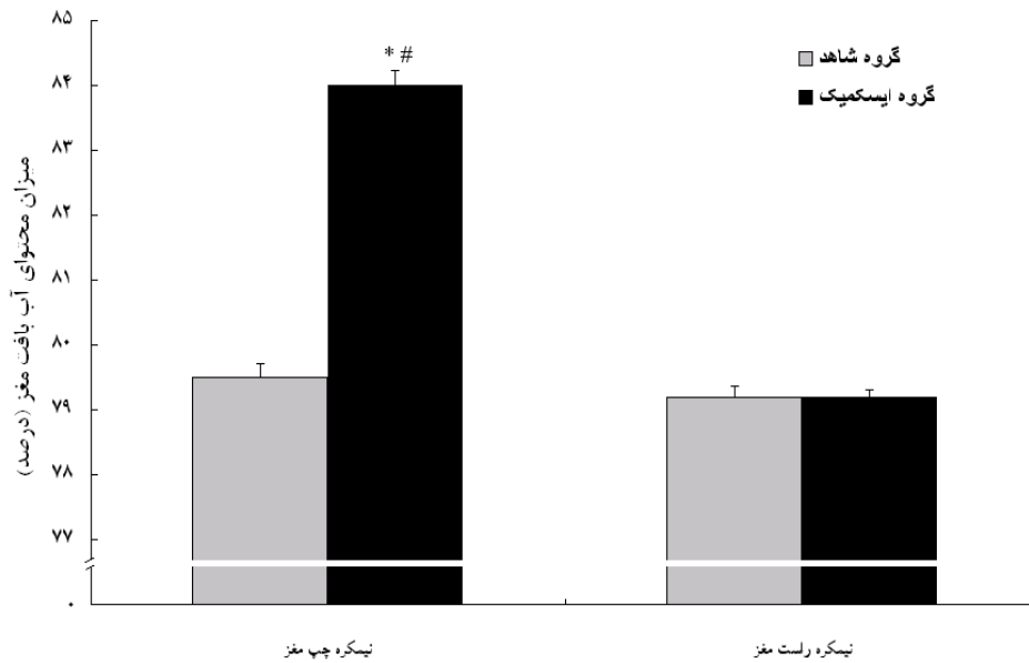
نمودار ۵. محتوی آب بافت نیمکره های مغز در حیوانات گروه شاهد (n=8) و گروه ایسکمیک (n=8)، ۲۴ ساعت پس از وقوع ایسکمی مغزی (* نسبت به نیمکره چپ گروه شاهد، # نسبت به نیمکره راست همانگروه، p < 0.05 ).
