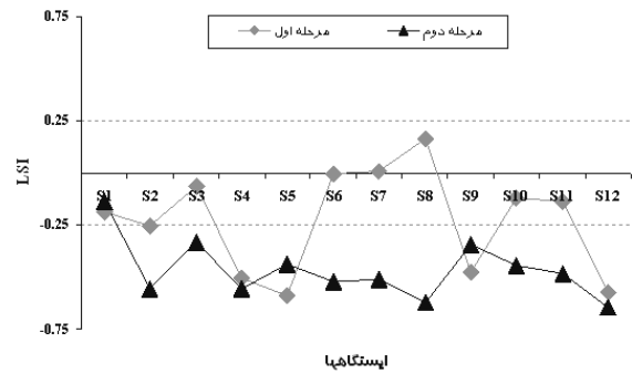
شکل ۱. مقایسه مقادیر شاخص اشباع لانژیه (LSI) در شبکه آب مشروب شهر اردبیل
