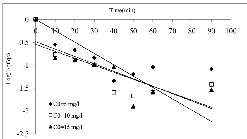
شکل ۵. منحنی سنتیک جذب بر اساس مدل شبه درجه اول برای جذب کروم
