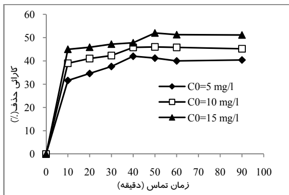
شکل ۲. تأثیر زمان تماس بر روی کارایی حذف Cr(VI) (غلظت اولیه ۵، ۱۰، ۱۵، دوز جاذب ۱g/L، pH=۵)
