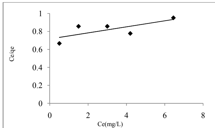
شکل ۷. نمودار \frac{C_e}{q_e} به صورت تابعی از C_e و معادله مشتق از آن بر اساس معادله لانگمیر
