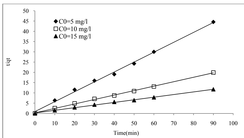
شکل ۶. منحنی سنتیک جذب بر اساس مدل شبه درجه دوم برای جذب کروم
