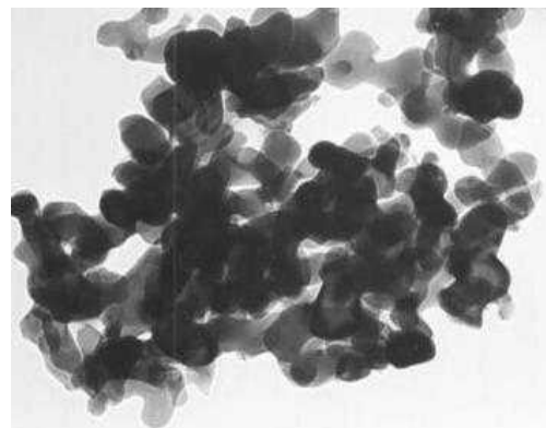
شکل ۱. عکس TEM از نانو ذره آلومینا
