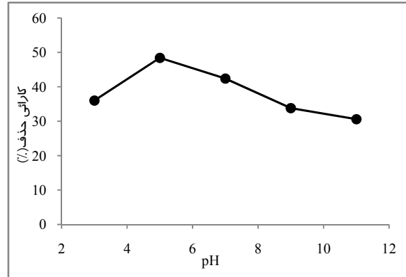
شکل ۴. بررسی تأثیر pH بر روی کارایی حذف کروم (در حضور ۰/۵ گرم جذب در ۵۰۰ سی سی نمونه با غلظت ۵ mg/l)
